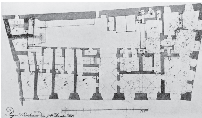
Půdorys Saského domu z roku 1826 (sever dole)
