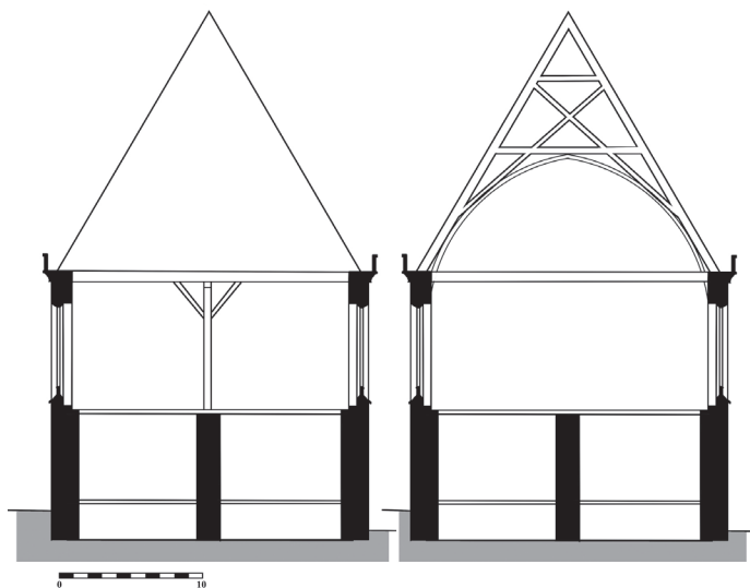
Saský dům, pokus o rekonstrukci prostorového uspořádání prvního patra s velkým sálem, vlevo varianta s rovným stropem, vpravo varianta s bedněnou klenbou.
