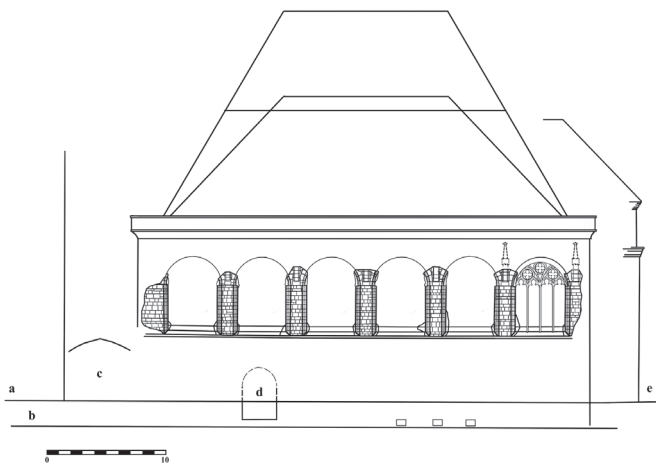
Saský dům, pokus o rekonstrukci severního průčelí paláce: a) dnešní úroveň terénu b) středověká úroveň terénu c) místo brány do dvora d) hlavní vstup do domu e) srovnání s dnešním stavem.
