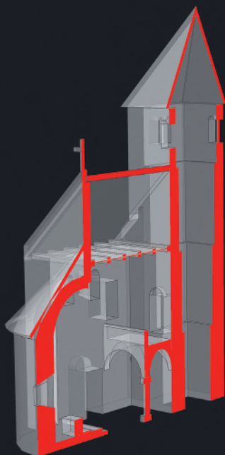
VELKÝ KOSTEL – řez
