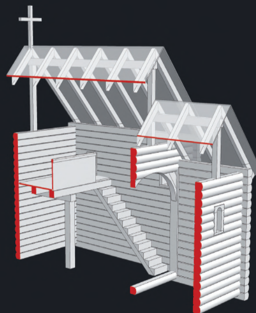
MALÝ KOSTEL – řez
